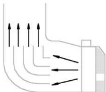
Рис. 5.2. Направление воздуха от радиатора отклоняющими лопастями
