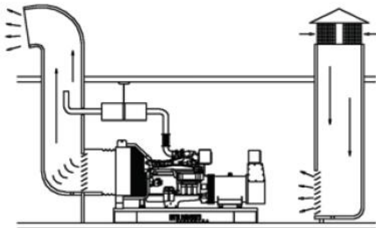
Рис. 5.4. Воздушная вентиляция
