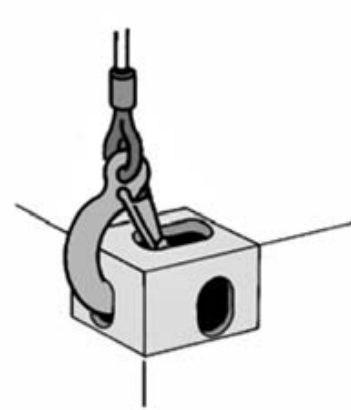
Пример захвата крюком с предохранительной скобой
