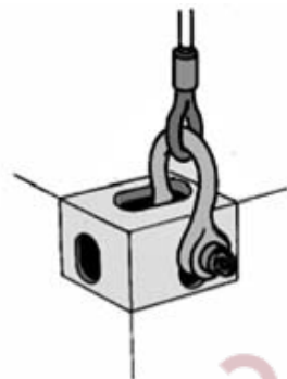
Пример подъема за скобу
