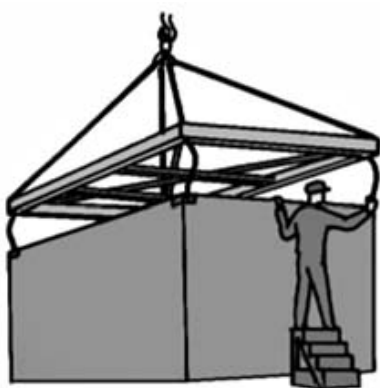
Крепление подъемного устройства
