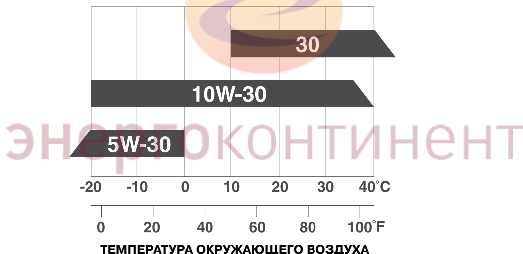
Температурный диапазон применимости масел по классификации SAE
