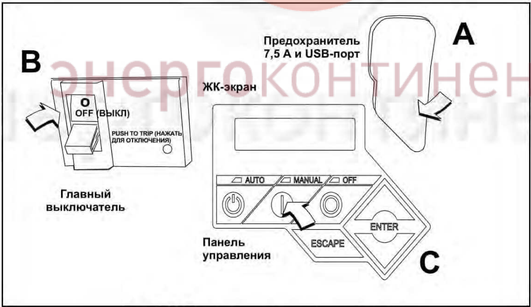
Рис. 3-5. Панель управления генератора
