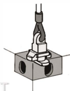
Пример подъема за замок, закрываемый вручную
