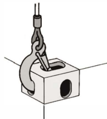
Пример захвата крюком с предохранительной скобой
