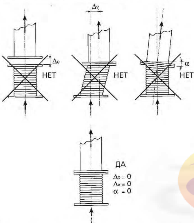
Рисунок 6-Е. Правильная сборка компенсирующего стыка.
