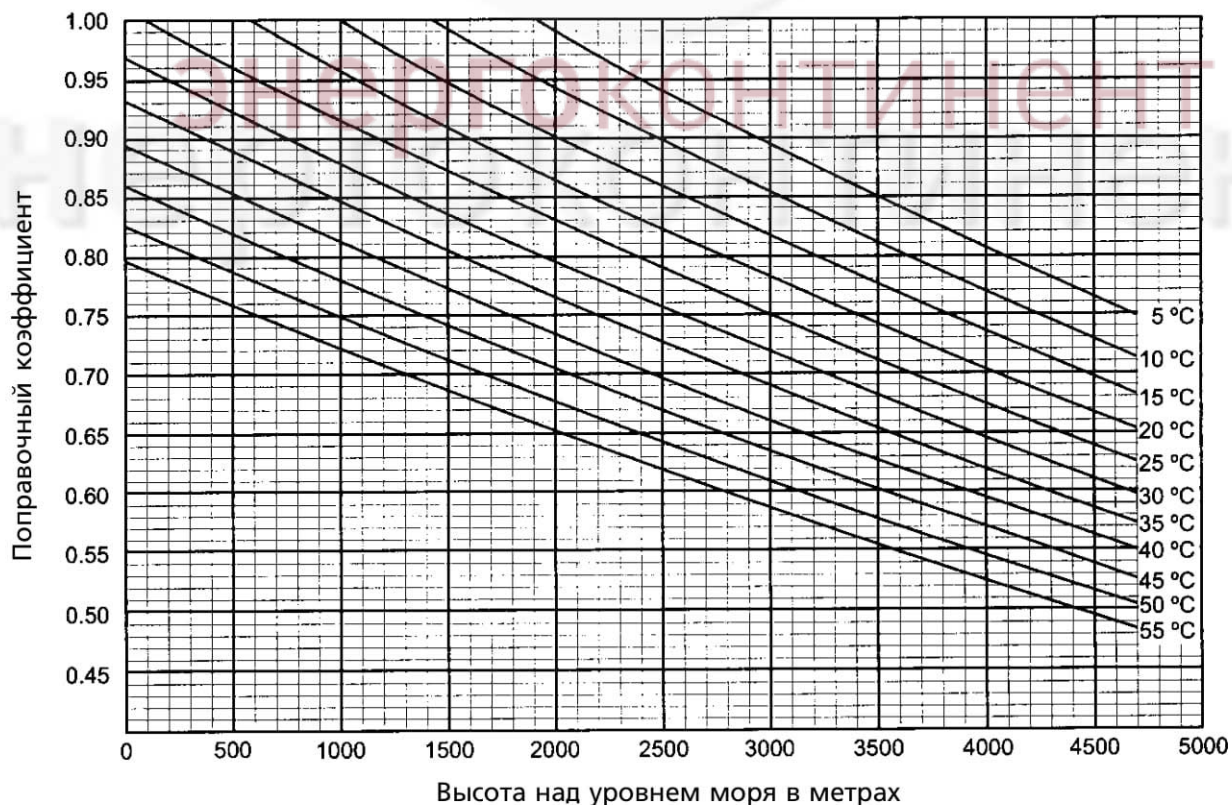
Рисунок 2-В. Коэффициенты изменения мощности двигателей с наддувом и промежуточным охладителем в зависимости от условий окружающей среды.
