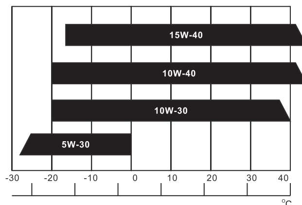
Степень вязкости SAE
