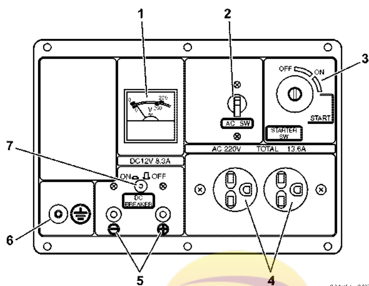
Панель (типовая)
