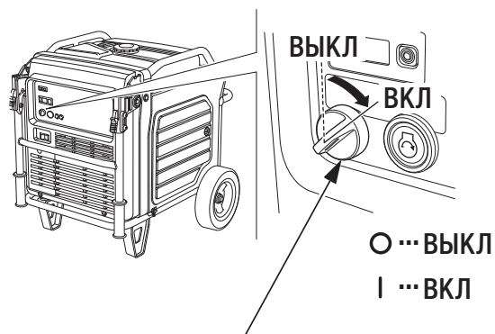
ВЫКЛЮЧАТЕЛЬ ЗАЖИГАНИЯ
