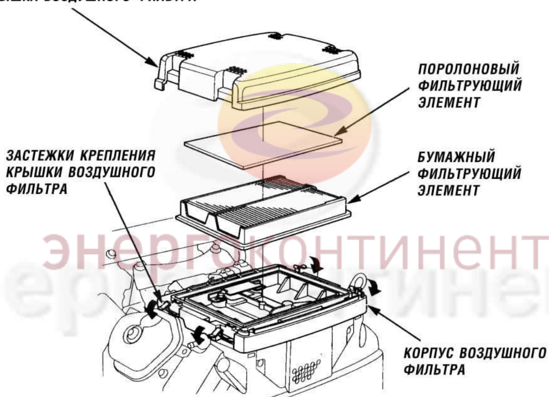
КРЫШКА ВОЗДУШНОГО ФИЛЬТРА
