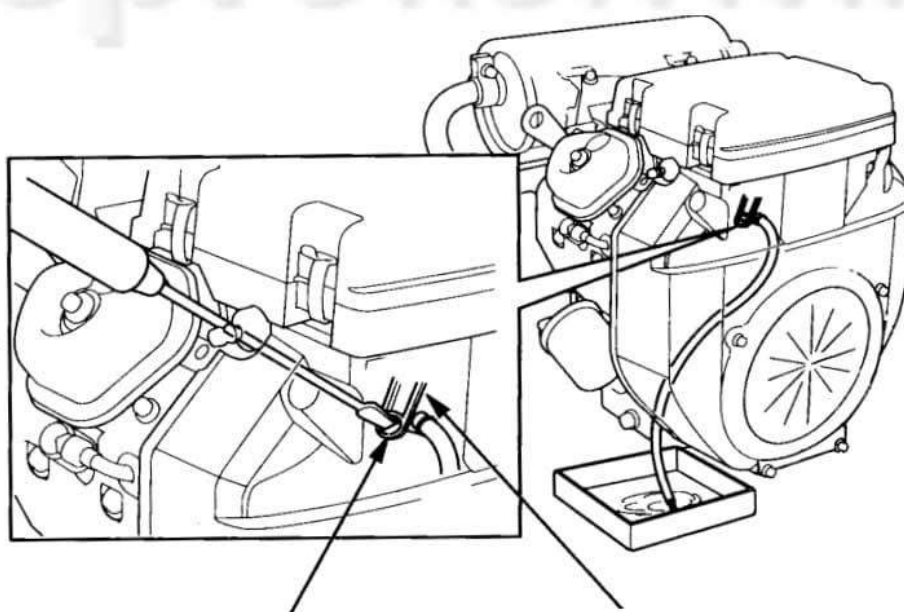
ЗАГЛУШКА СЛИВНОГО ОТВЕРСТИЯ
