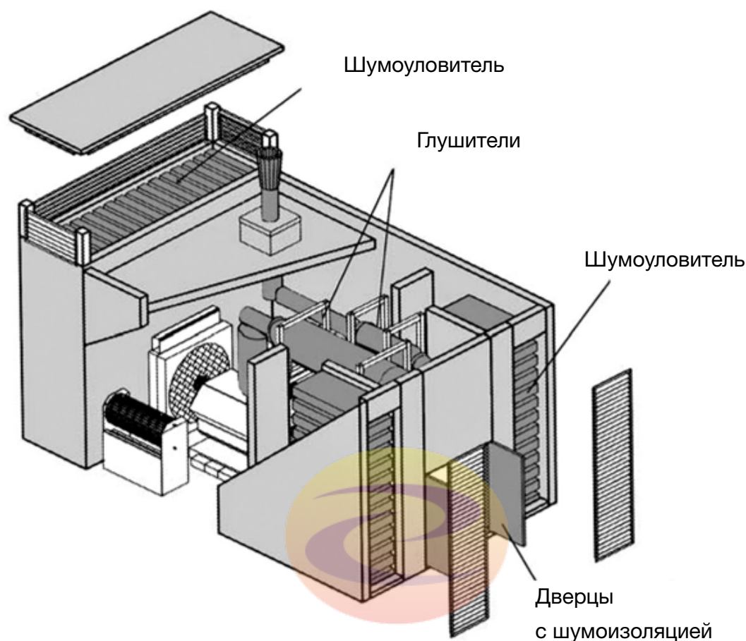
Пример установки
