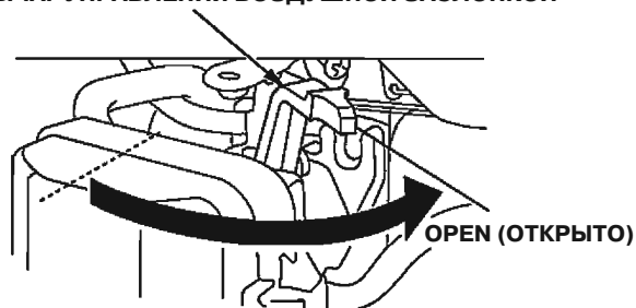
РЫЧАГ УПРАВЛЕНИЯ ВОЗДУШНОЙ ЗАСЛОНКОЙ
