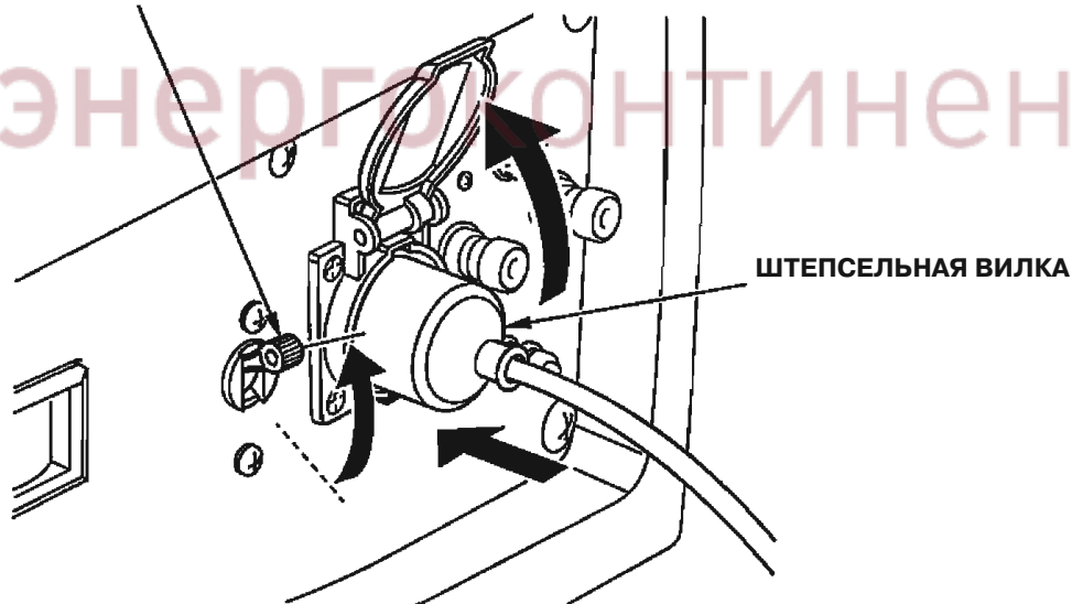
ПРЕРЫВАТЕЛЬ ЦЕПИ ПЕРЕМЕННОГО ТОКА
