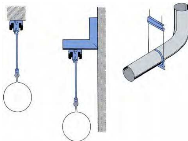
Рисунок 2.18: Подвеска
