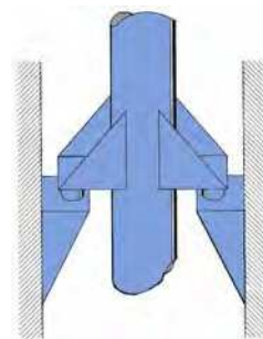
Рисунок 2.20: Опоры колонны
