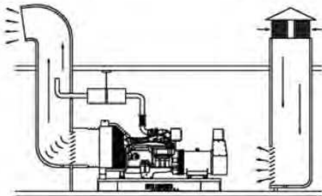
Рис. 12.3 - Воздушная вентиляция
