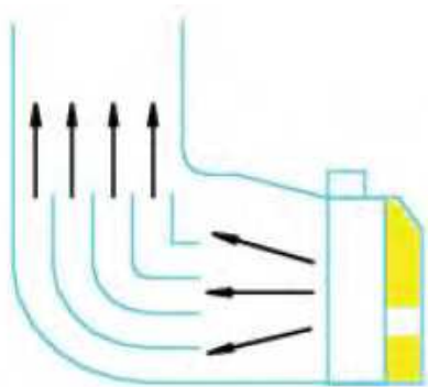
Рис. 12.1 - Направление воздуха от радиатора отклоняющими лопастями
