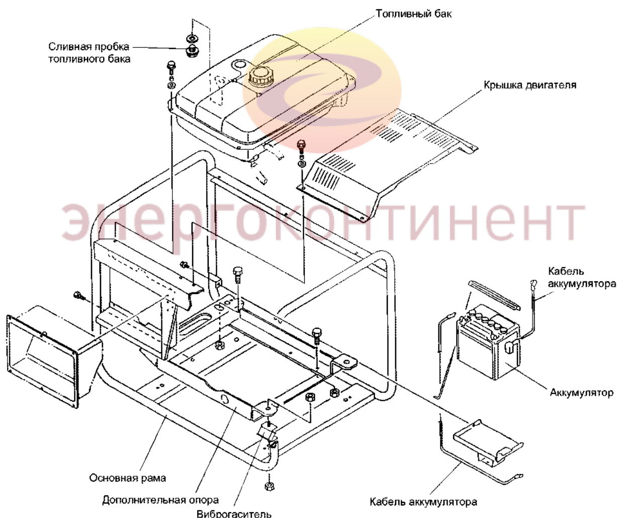
Рис. 4 Рама
