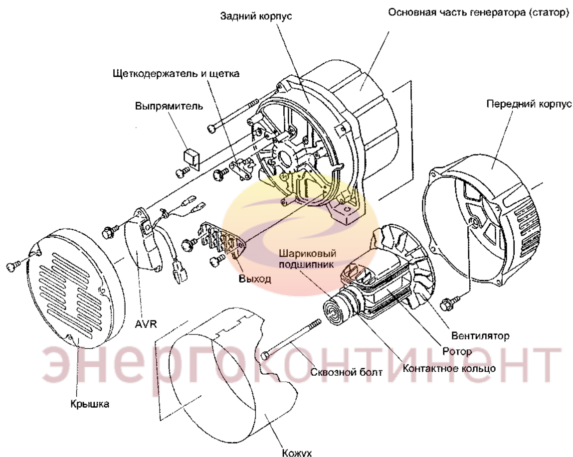
Рис. 6 Блок генератора
