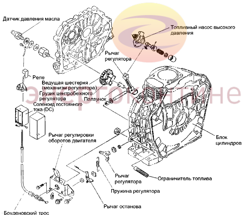
Рис. 11 Система управления
