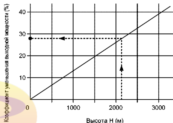
Рис. 47 Высота — уменьшение выходной мощности
