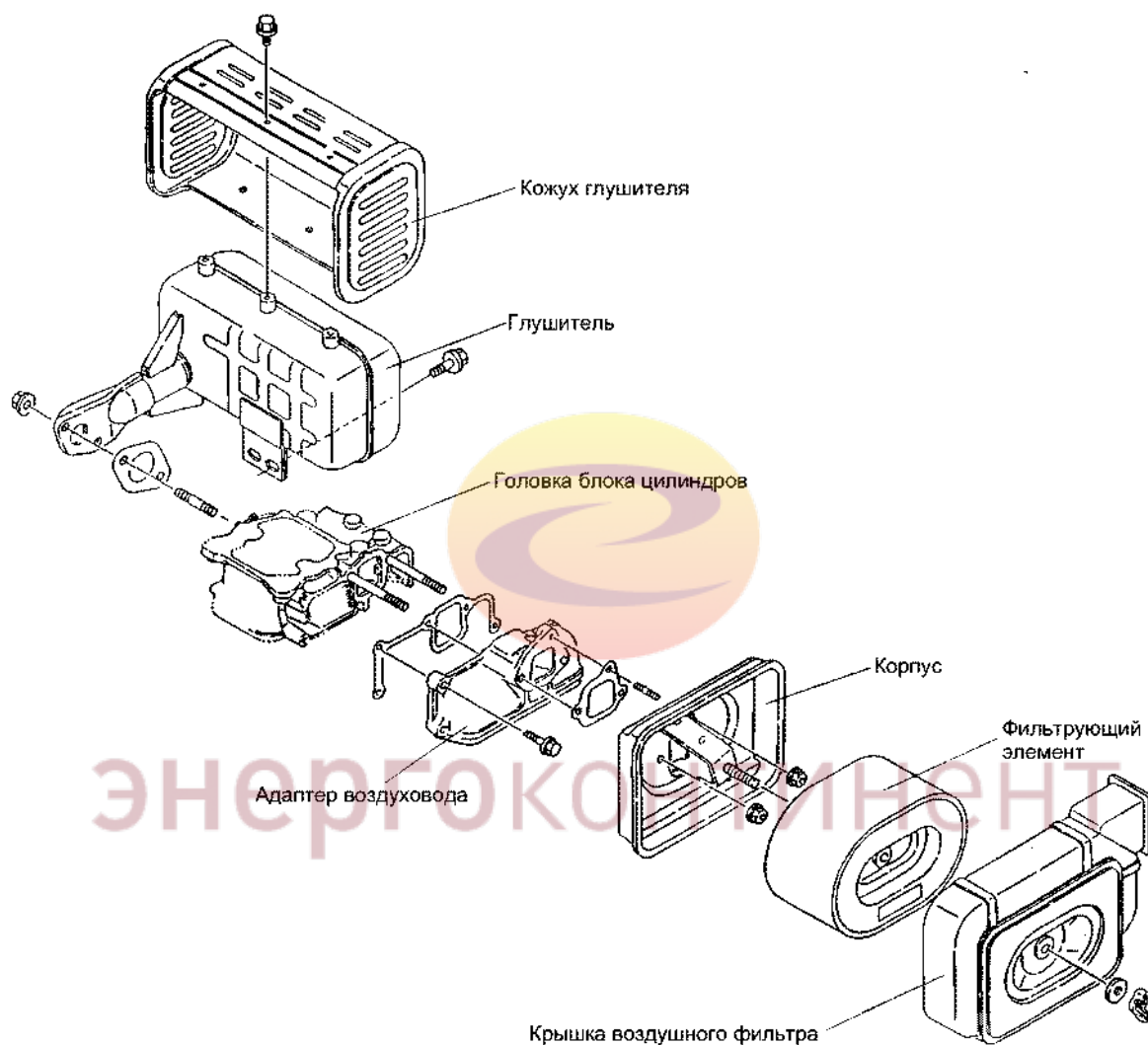
Рис. 8 Система подачи воздуха и выхлопная система
