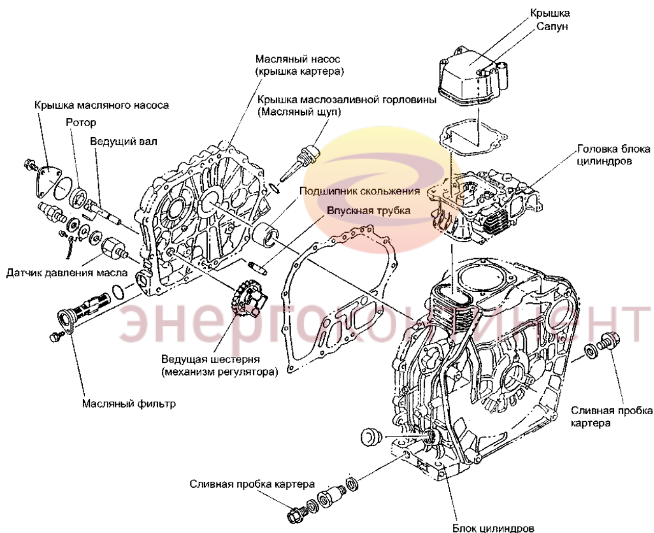
Рис. 9 Система смазки
