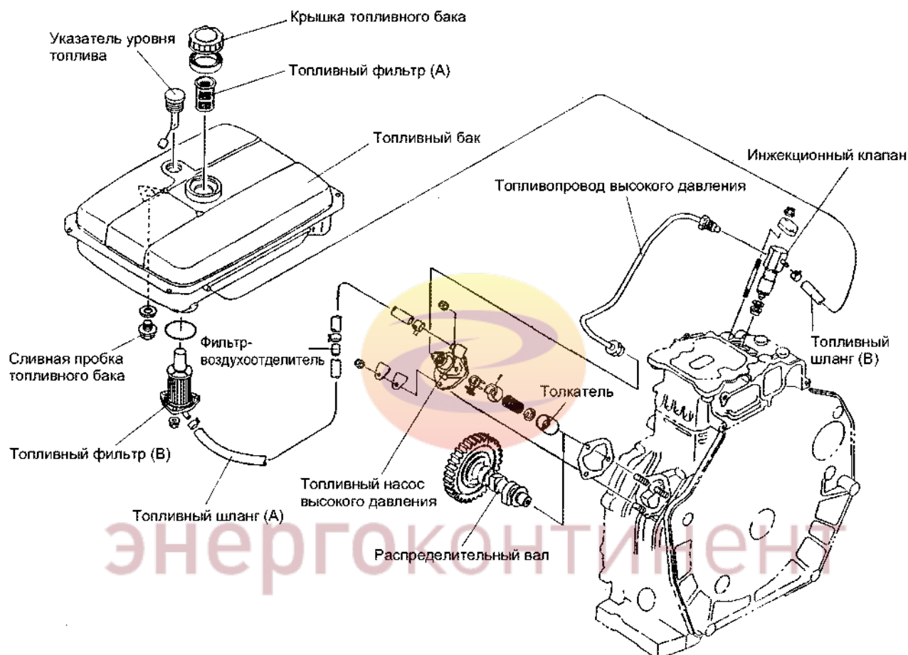
Рис. 10 Топливная система
