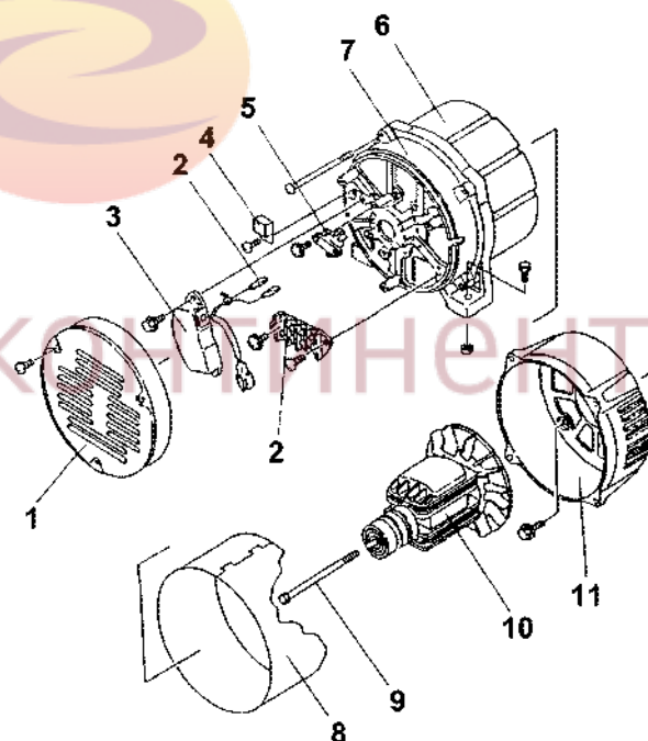
Рис. 15 Компоненты блока генератора
