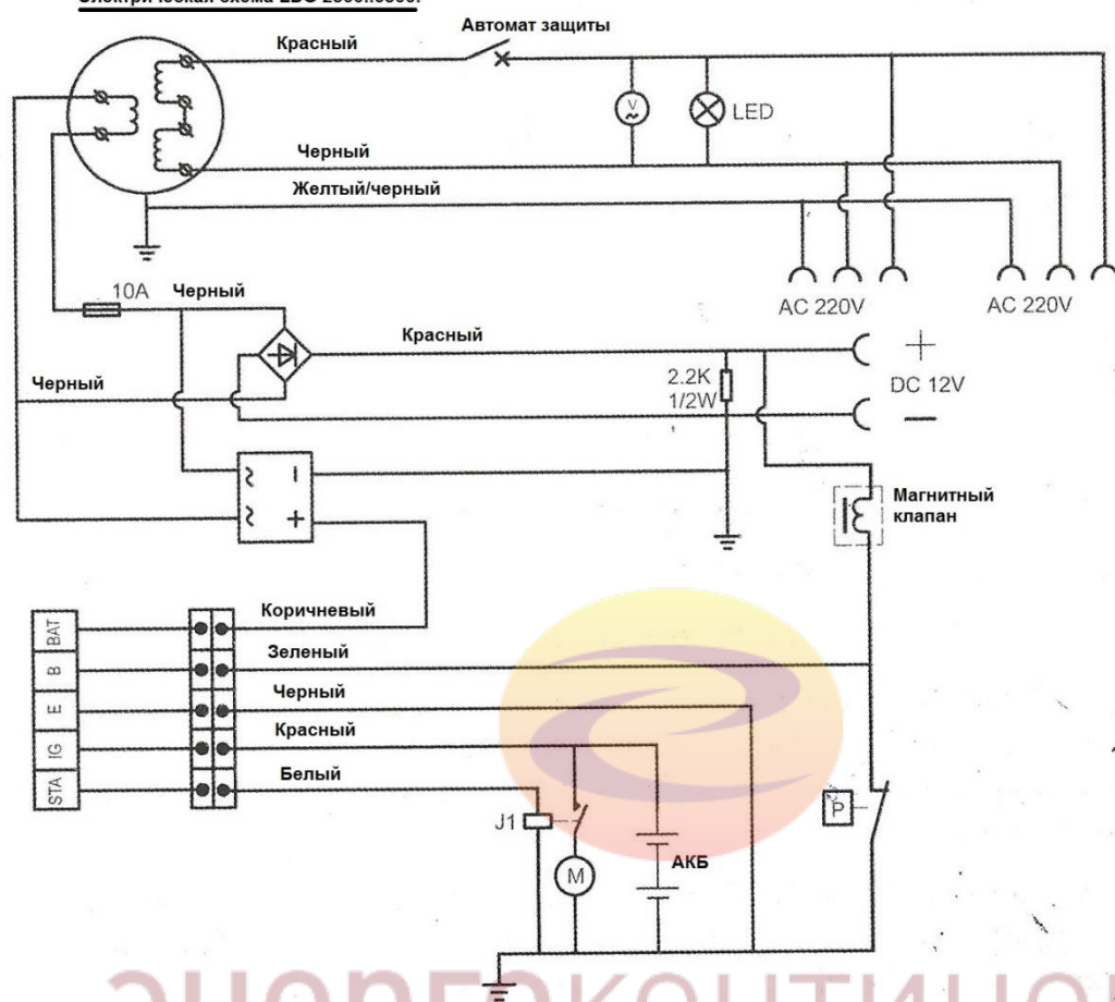
Стартерный замок
